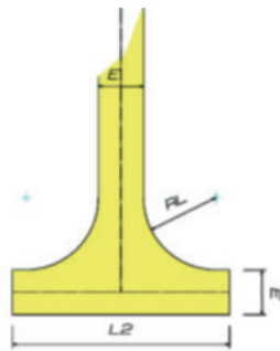
AIRE DE RETOURNEMENT « EN T »
