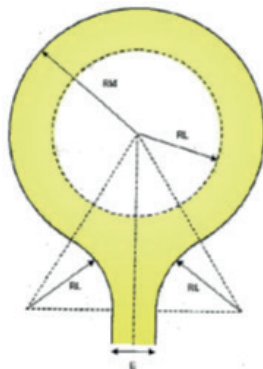
AIRE DE RETOURNEMENT « GIRATOIRE »
