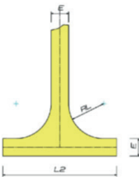
AIRE DE RETOURNEMENT « EN L »
