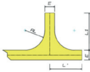
AIRE DE RETOURNEMENT « EN L »
