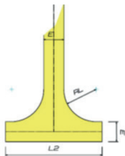
AIRE DE RETOURNEMENT « EN T »
